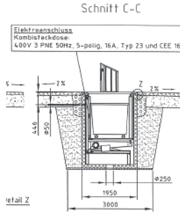
Schnitt C-C
