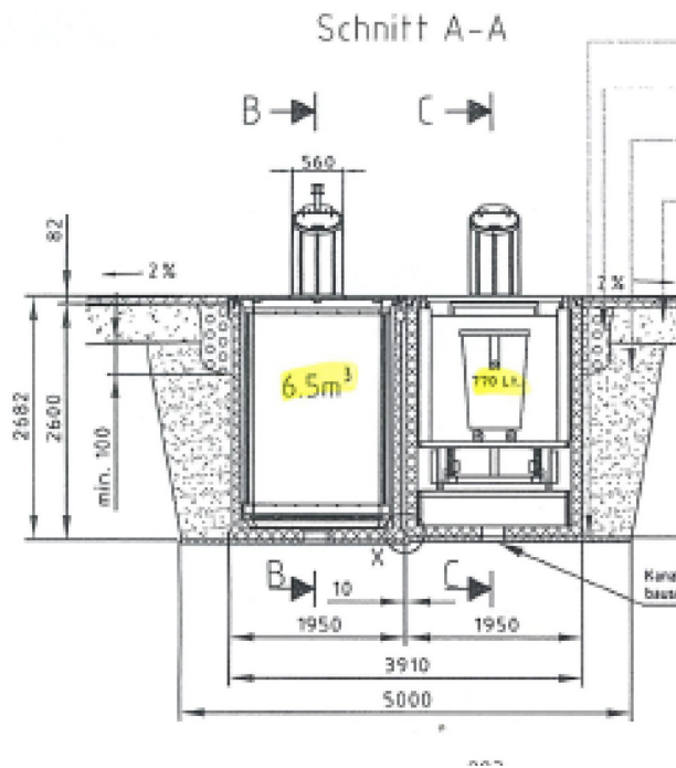
Schnitt A-A
