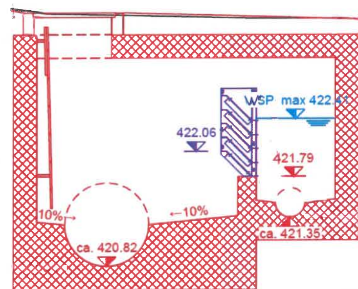
Schnitt A-A
